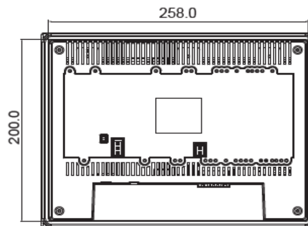
背視圖
