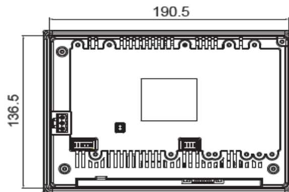
開孔尺寸
