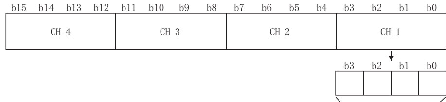
输入类型的设置内容
