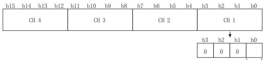
偏置·增益设置的设置内容
