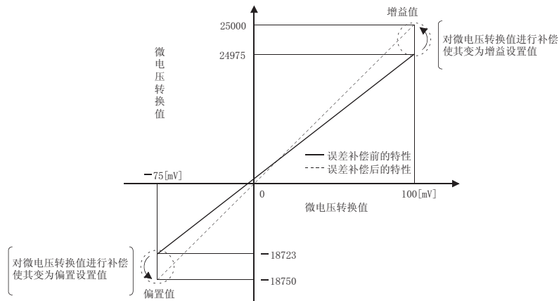
(b) 微电压输入时
