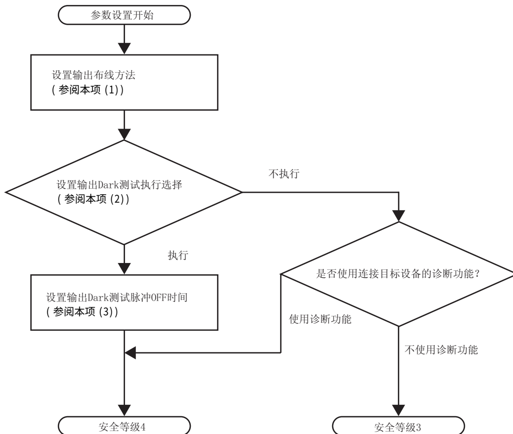
图 5.12 输出参数设置流程
