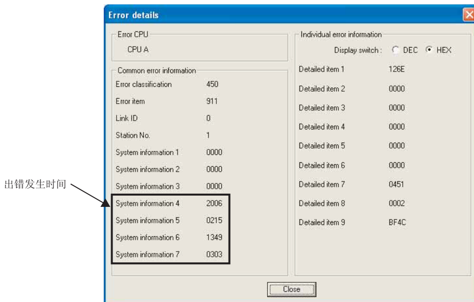
图 9.12 出错详细画面
