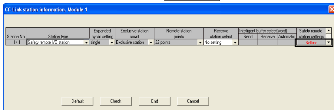
图 5.3 站信息设置画面
