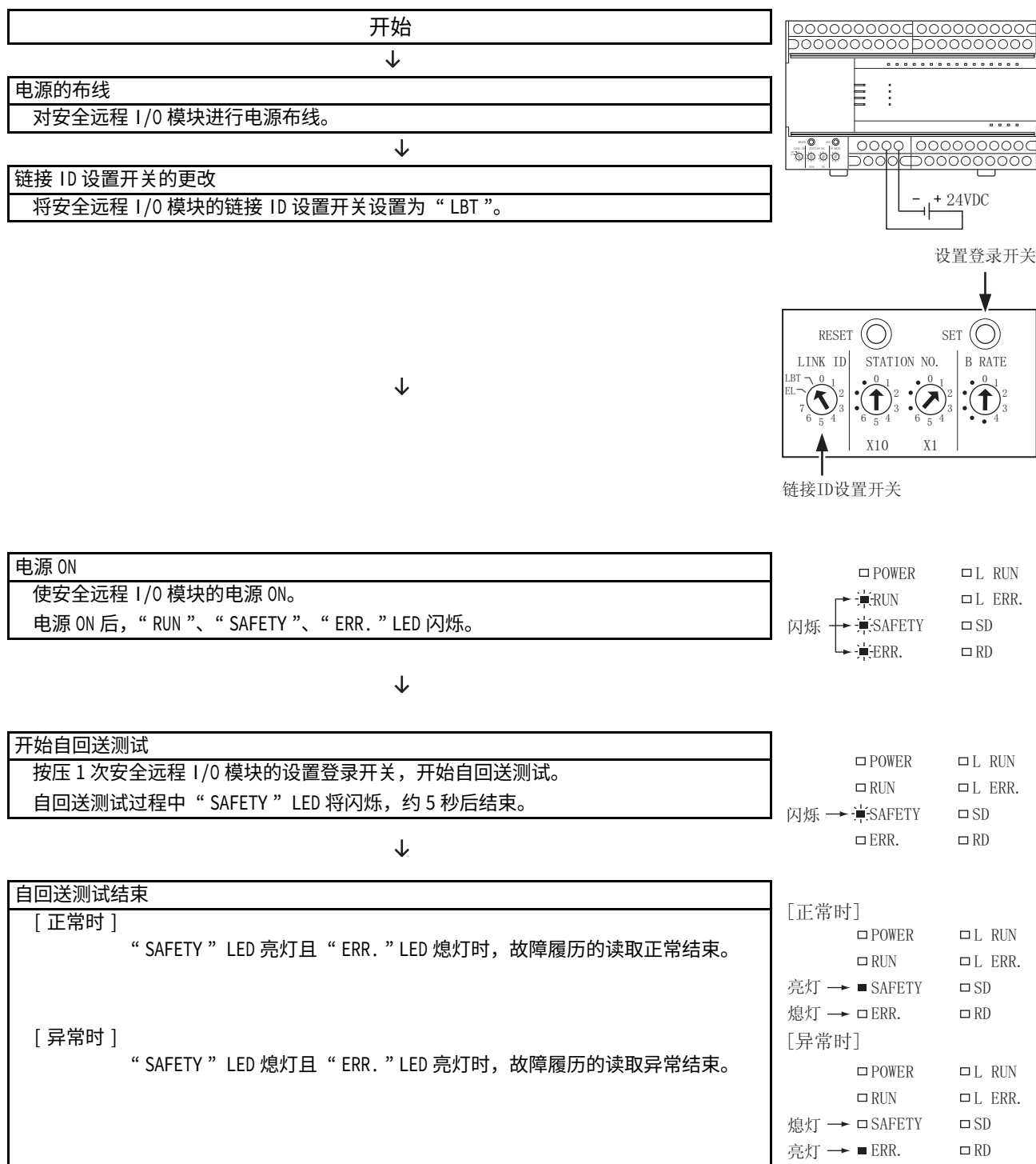
图 6.6 自回送测试执行步骤
