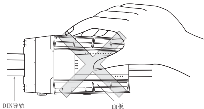
图 6.4 DIN 导轨的安装
