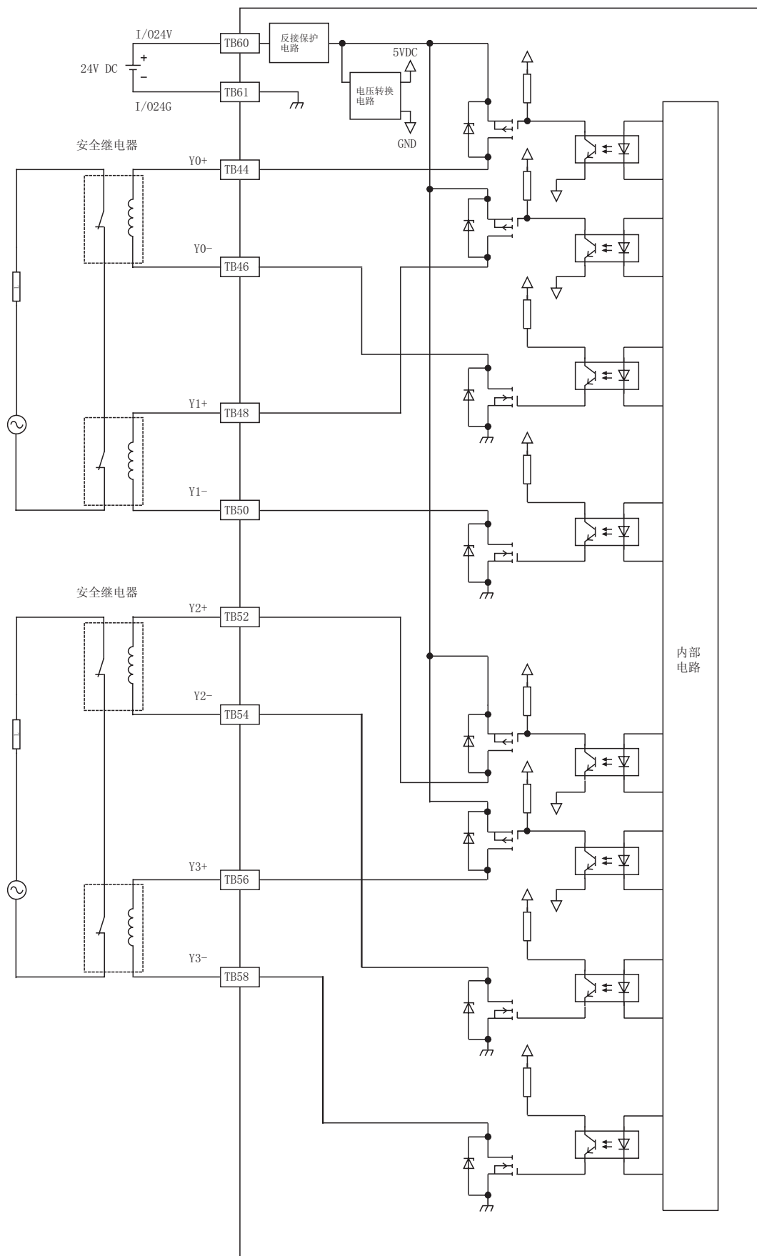
图 6.12 与输出设备的布线示例
