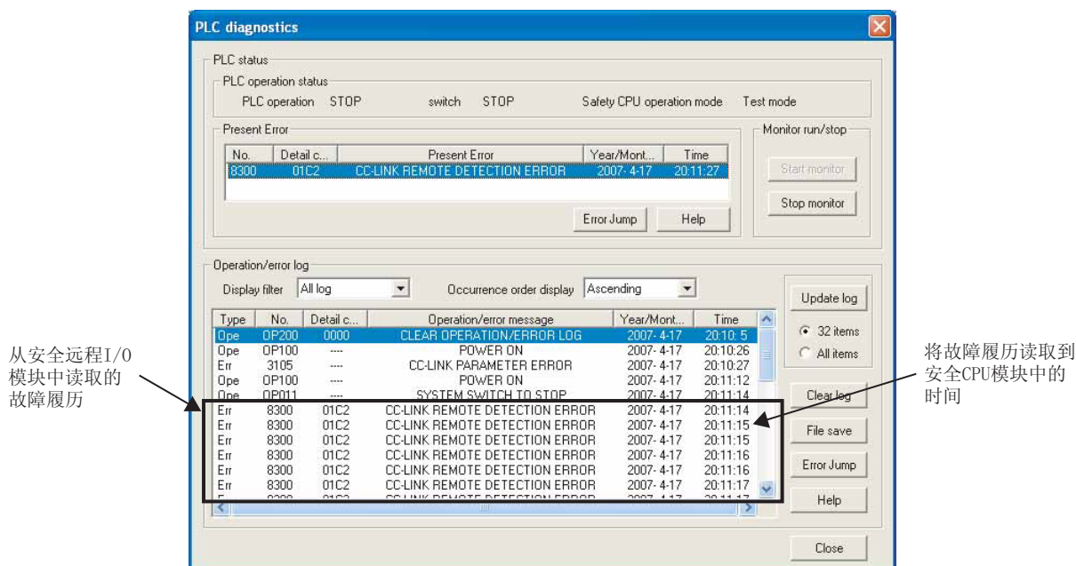
图 9.11 故障履历的显示
