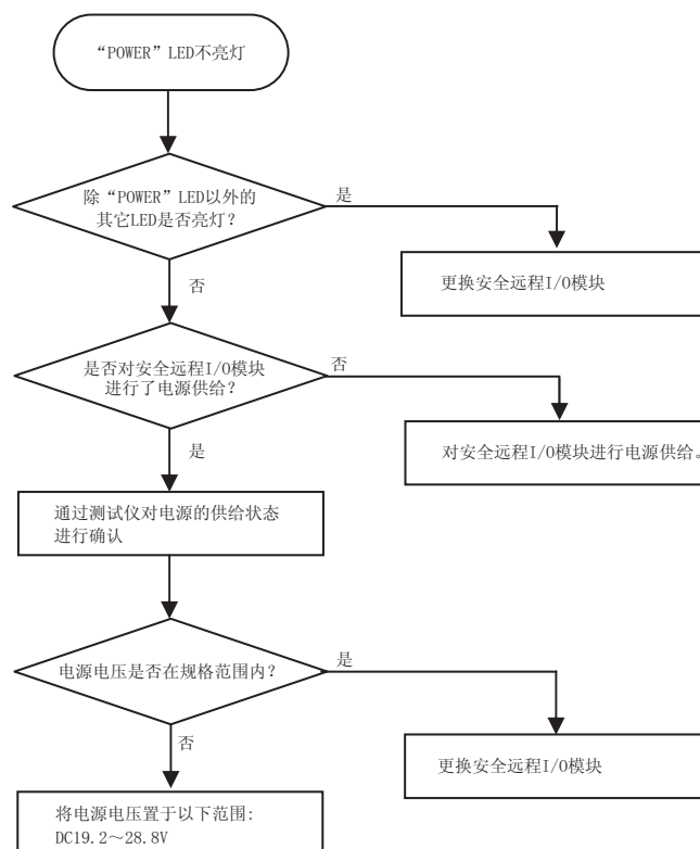
图 9.2 “POWER” LED 不亮灯时的流程
