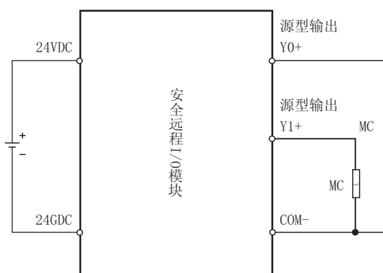
图 4.4 将源型输出与源型输出组合的冗余布线方法
