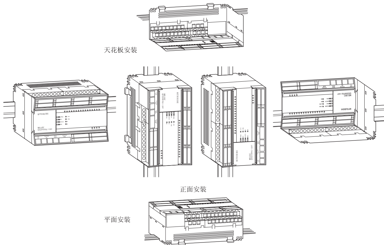
图 1.1 模块安装方向
