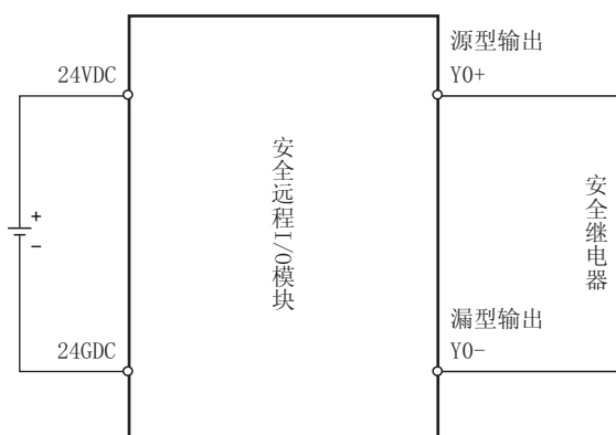
图 4.3 源型输出与漏型输出组合的冗余布线方法
