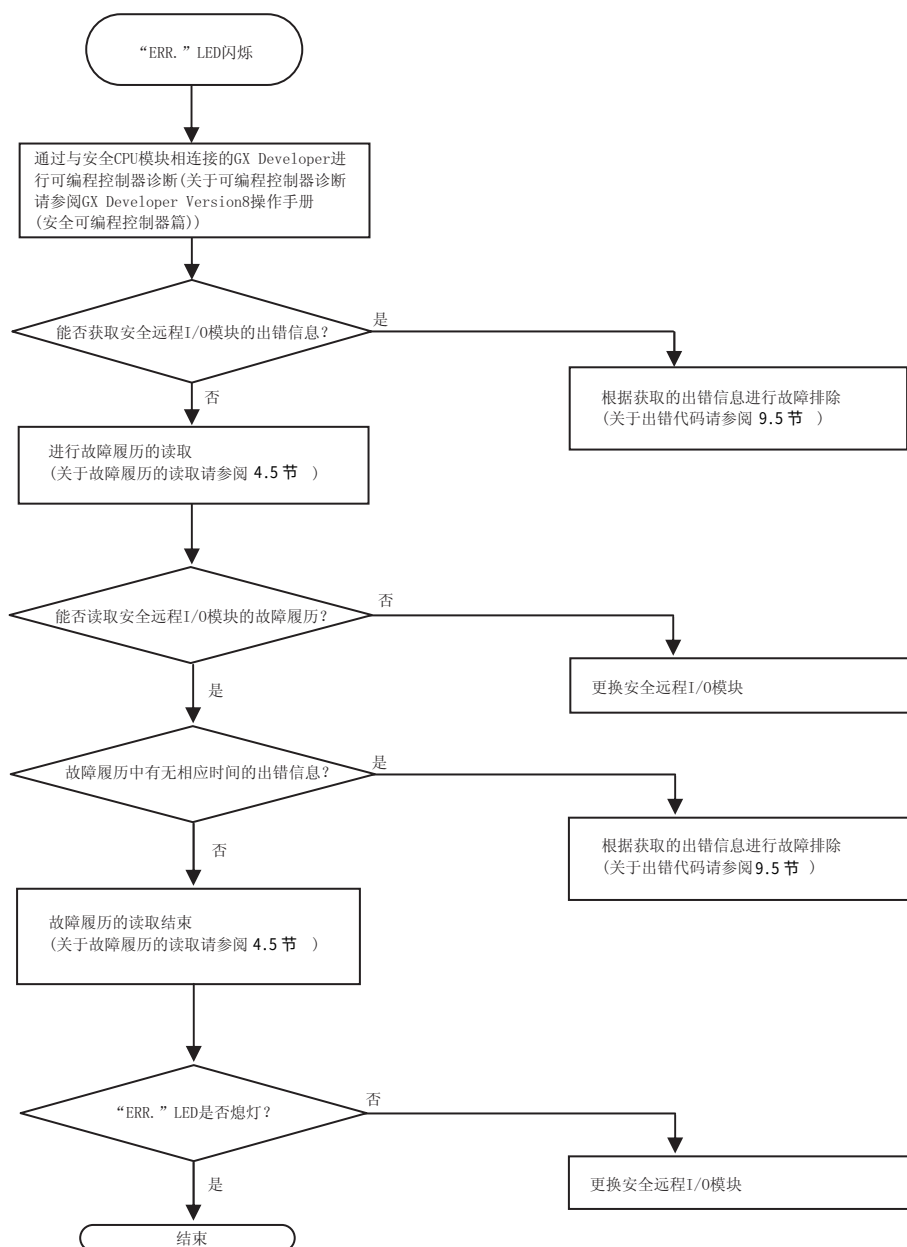
图 9.4 “ERR.” LED 闪烁时的流程
