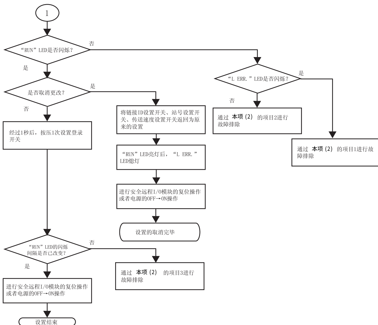
图 6.13 开关设置
