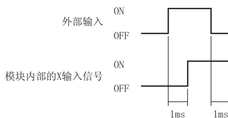
图 4.2 输入信号的延迟
