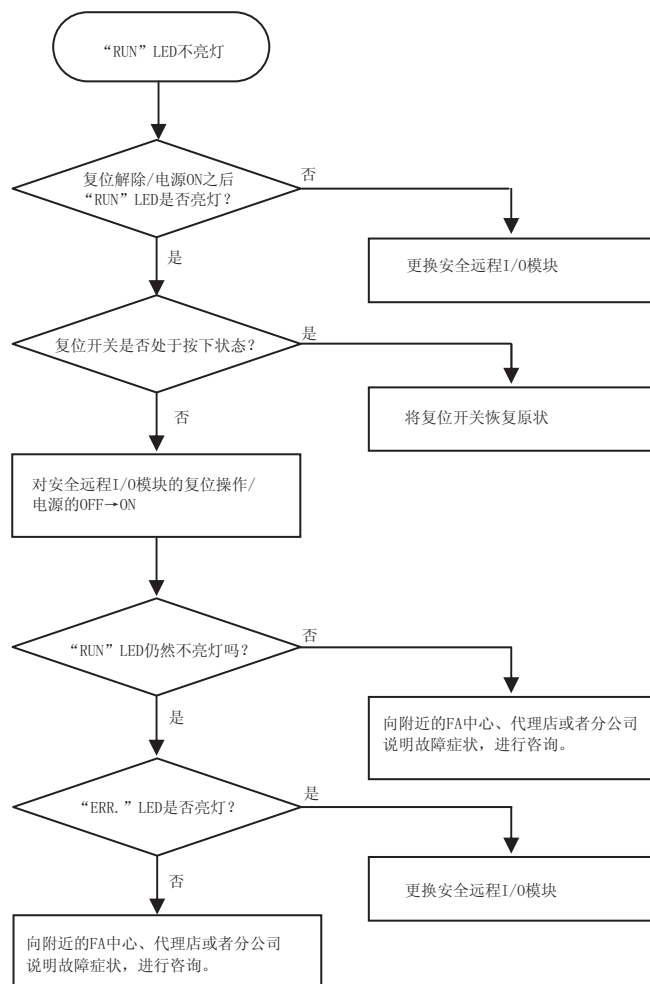
图 9.3 “RUN” LED 不亮灯时的流程
