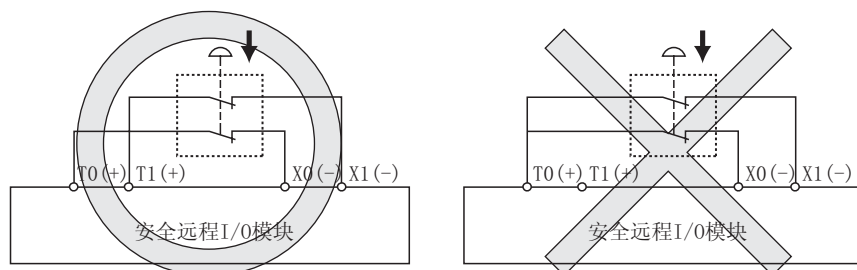
图 6.9 与测试脉冲端子的组合示例
