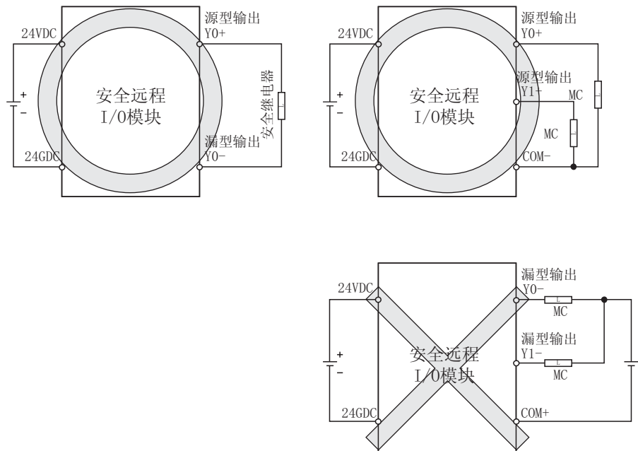
图 6.10 输出端子的组合示例
