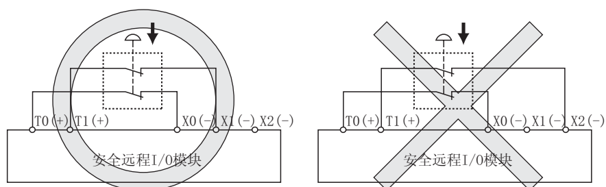
图 6.8 输入端子的组合示例
