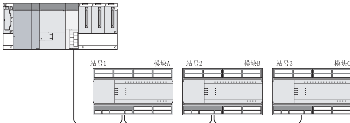
图 9.8 出错确认的配置示例
