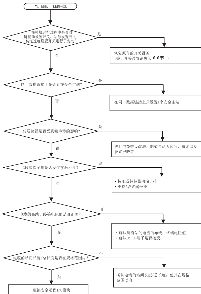
图 9.7 “L ERR.” LED 闪烁时的流程
