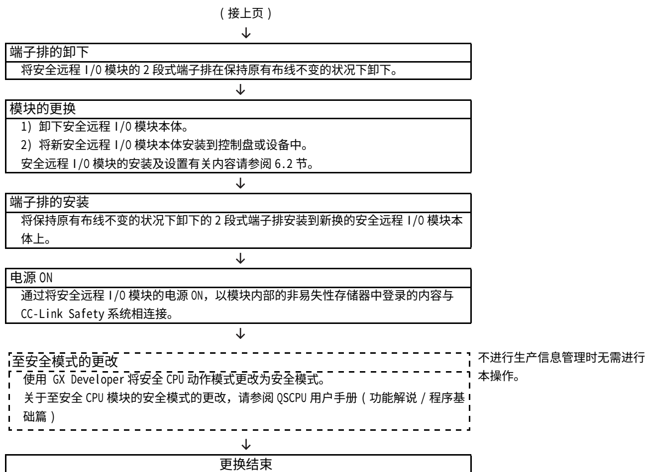
图 6.2 安全远程 I/O 模块的更换步骤
