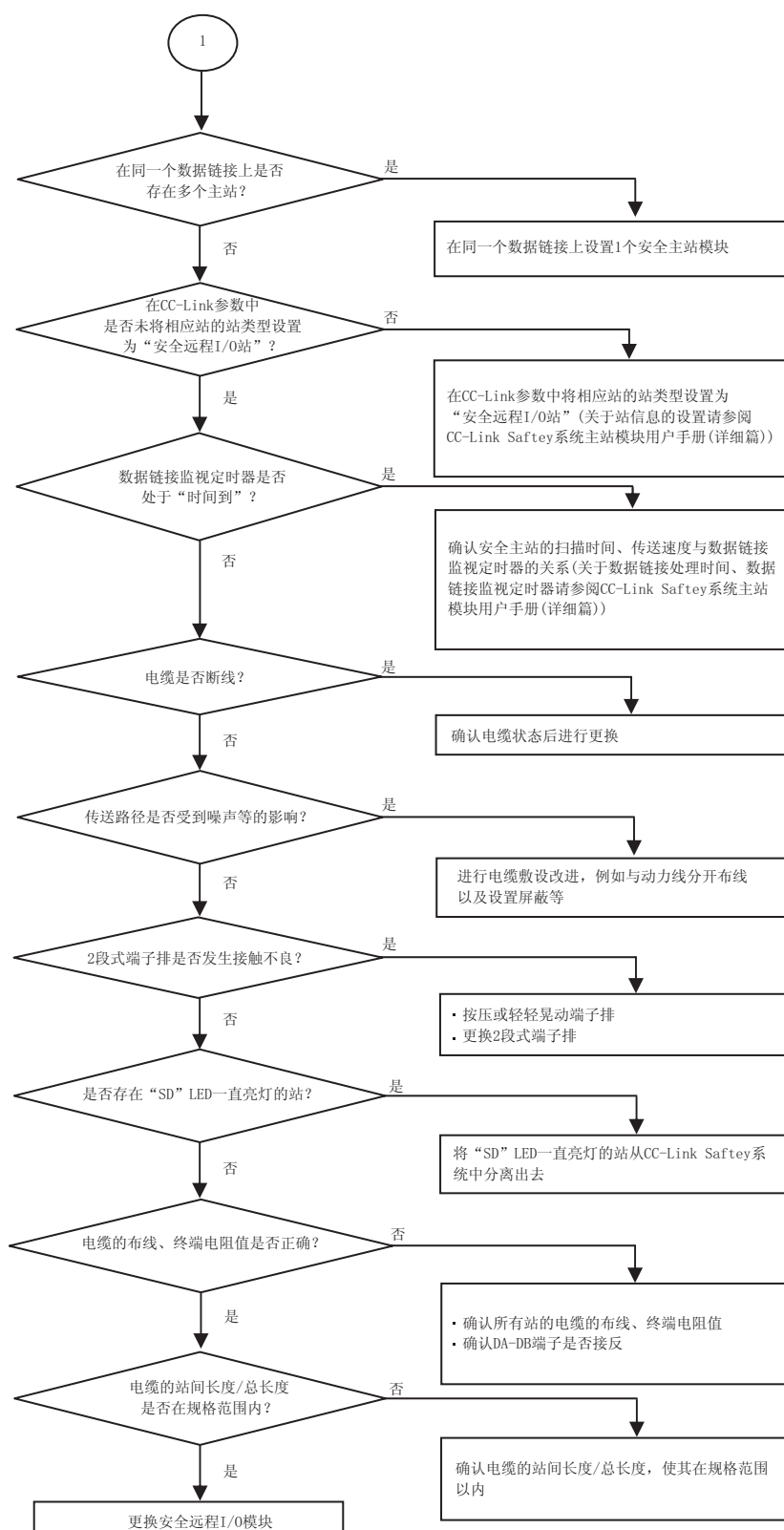
图 9.5 “SAFETY”LED 不亮灯时的流程
