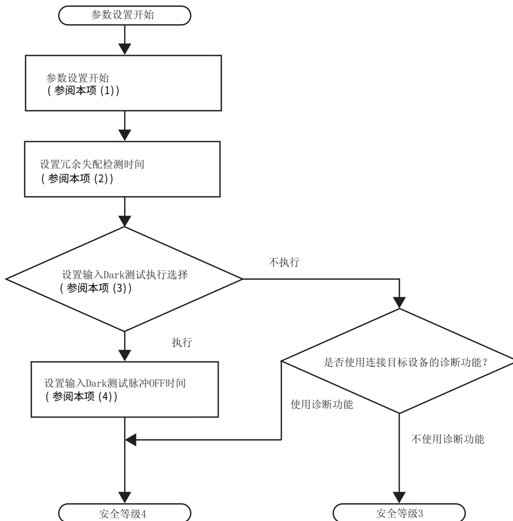
图 5.11 输入参数设置流程
