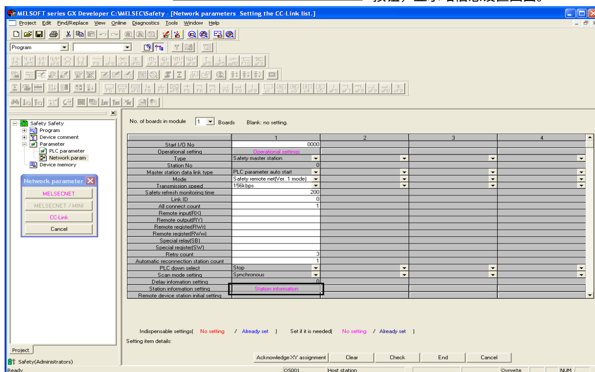
图 5.1 CC-Link 设置画面
