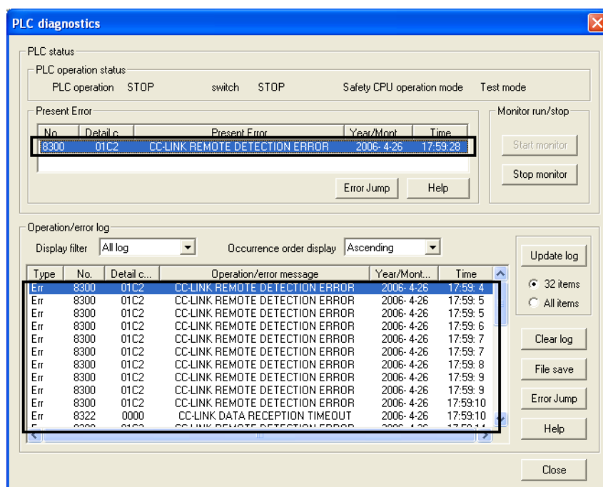
图 9.9 可编程控制器诊断画面
