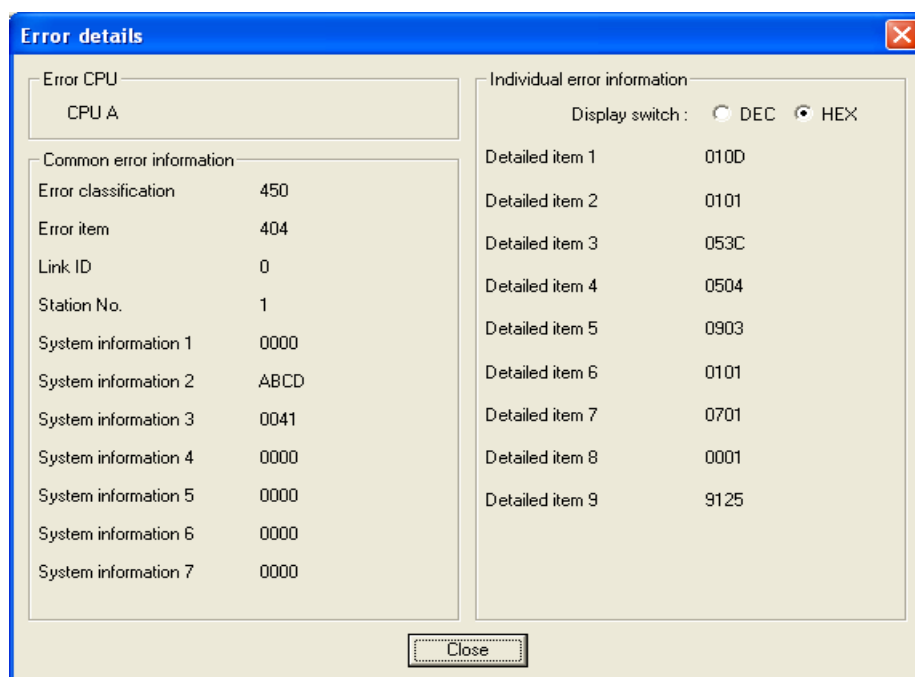
图 9.10 出错详细画面
