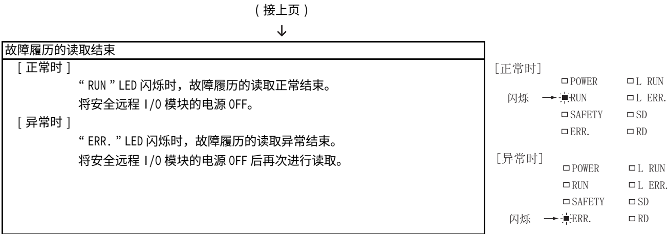
图 4.5 故障履历的读取步骤
