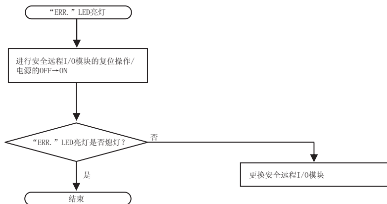
图 9.6 “ERR.” LED 亮灯时的流程
