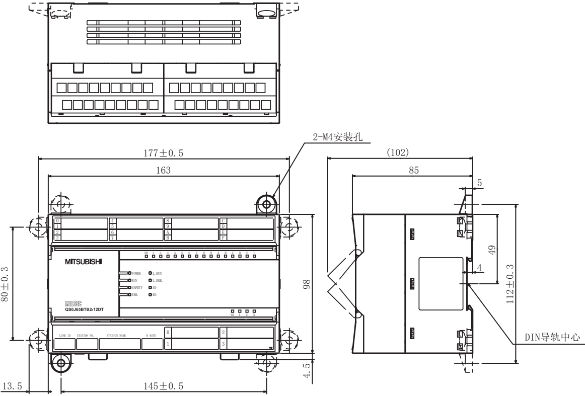
附图 1 外形尺寸图
