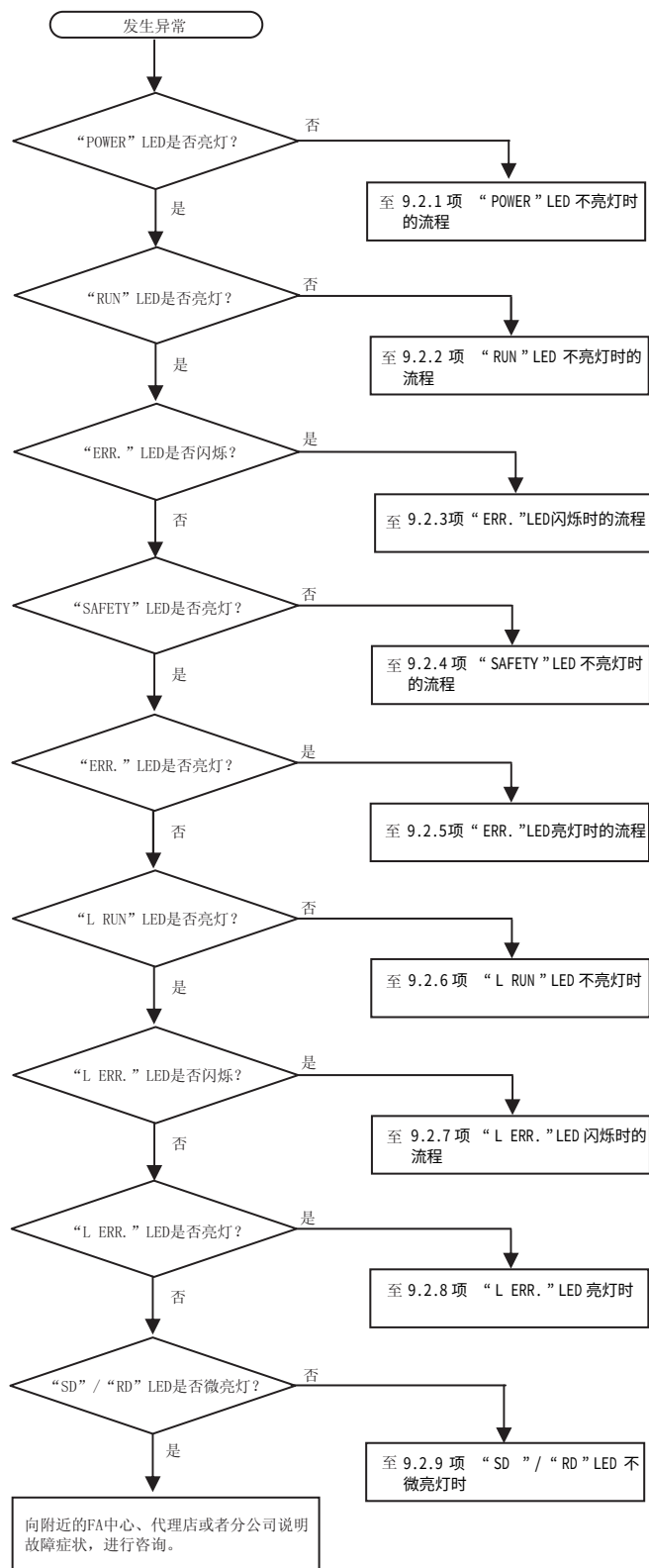
图 9.1 故障排除流程
