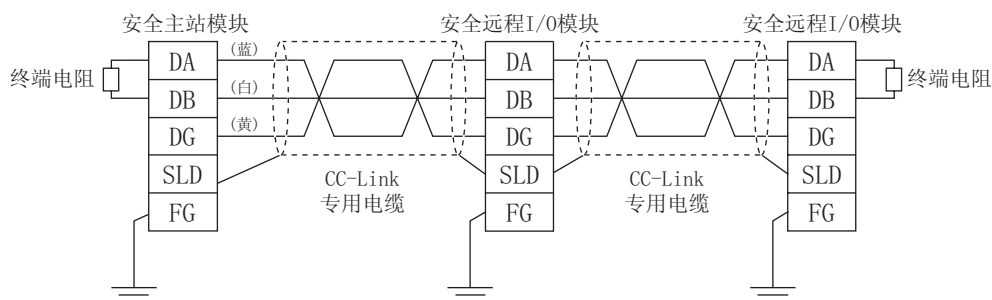
图 6.7 CC-Link 专用电缆连接
