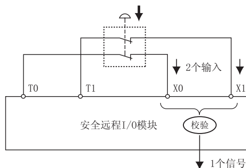
图 4.1 输入冗余布线
