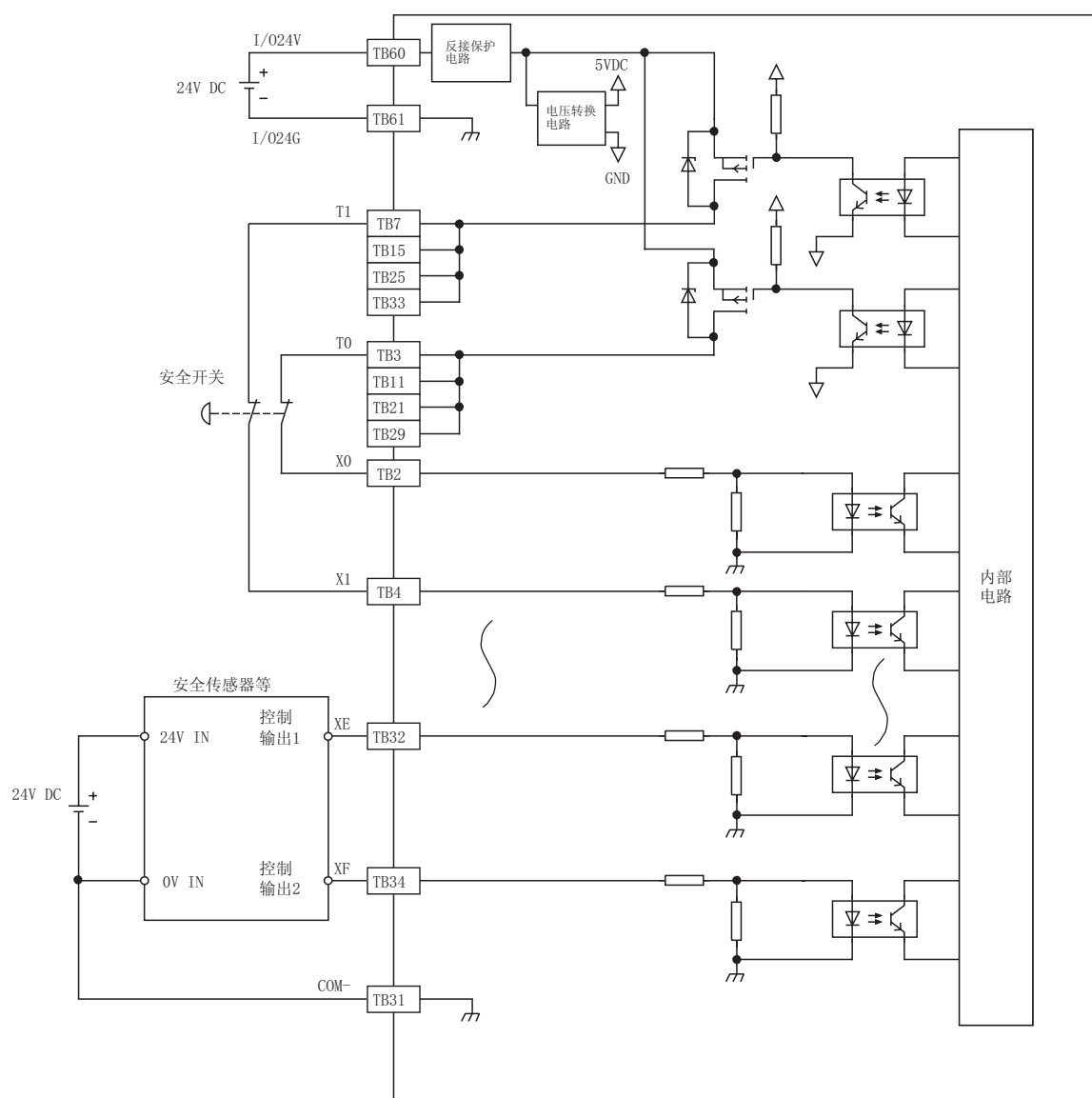
图 6.11 与输入设备的布线示例
