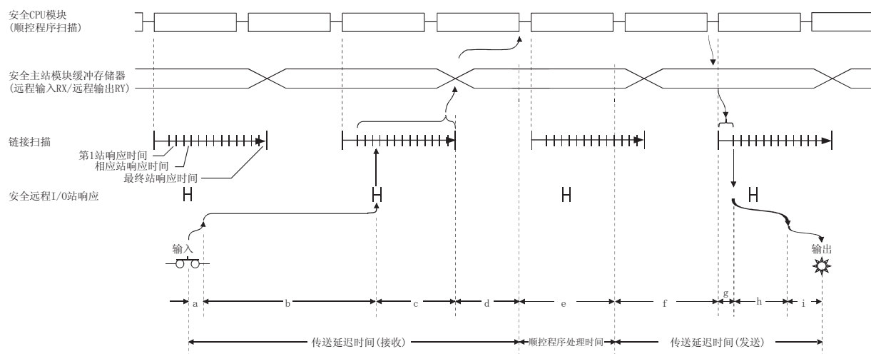
(b) 顺控程序扫描 &lt; 链接扫描时
