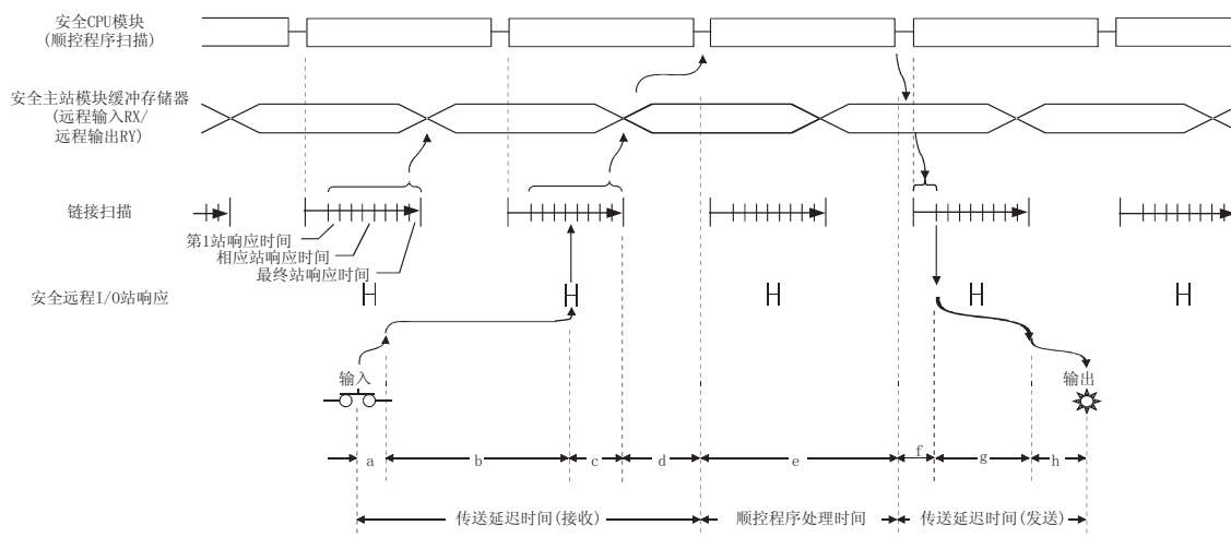
(a) 顺控程序扫描 \geq 链接扫描时
